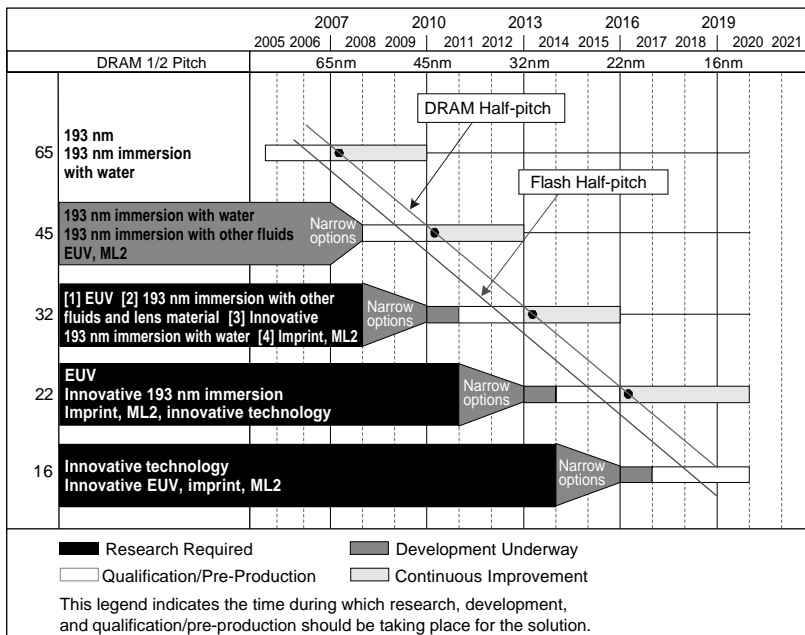
図4. リソグラフィ技術の候補
