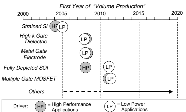
図6. MOSトランジスタの新規技術の導入時期
