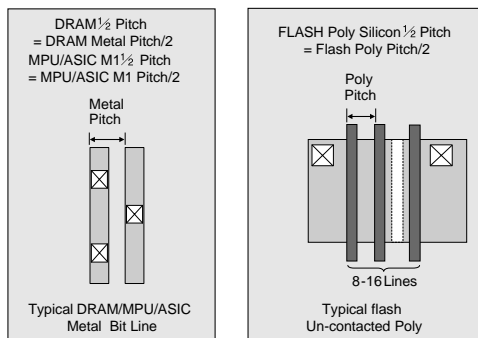
図 2. ハーフピッチの定義
