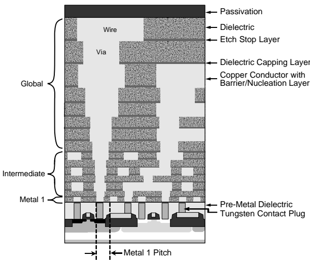
図8. 多層配線の断面構造とM1配線層の定義
