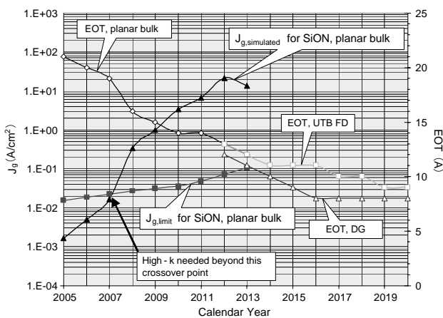
図5. ゲート絶縁膜のリーク電流とEOT（実効酸化膜厚）の推移 2008年以降、SiONでのリーク電流が大きくなり、High-kゲート絶縁膜が導入される。
