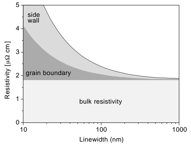
図9. Cu配線幅の縮小にともなう実効的な配線抵抗の上昇
