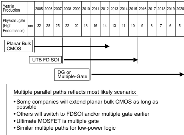
図7. 高性能 (High Performance) MOSFETのロードマップにおけるパラレルパス (parallel paths) 2008年以降、平面のバルクCMOSトランジスタ、FD-SOIのトランジスタ、マルチゲートのトランジスタなどが使われるが、用途により、また各社の戦略により、複数のトランジスタ構造が利用される。
